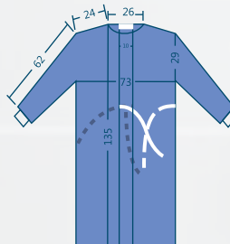
Gown
